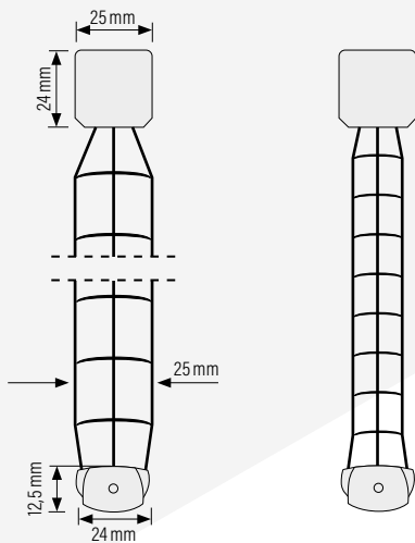
Standard-Jalousie 25 mm Lamellen
