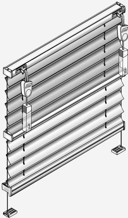
Profil Bedienschiene
